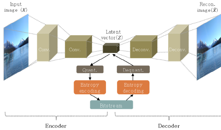
그림 1. 합성곱 오토인코더 기반 이미지 압축 개념 Fig. 1. The concept of image compression based on the convolutional autoencoder
