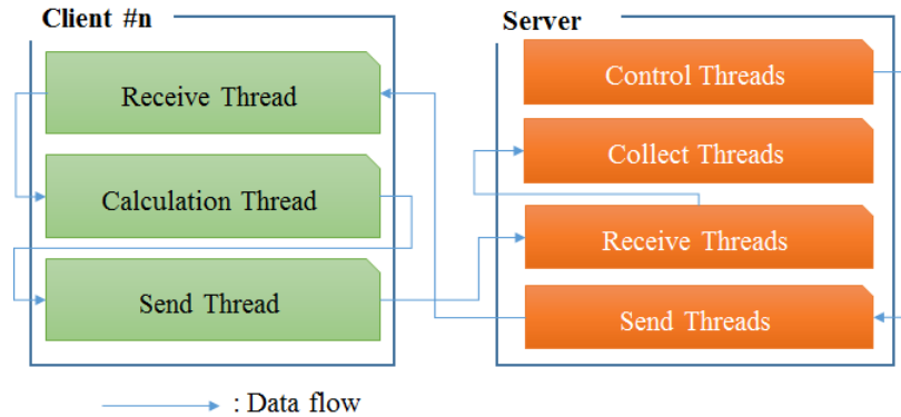
그림 3. 제안 방법의 프로그램 구조 Fig. 3. Program structure of the proposed method
