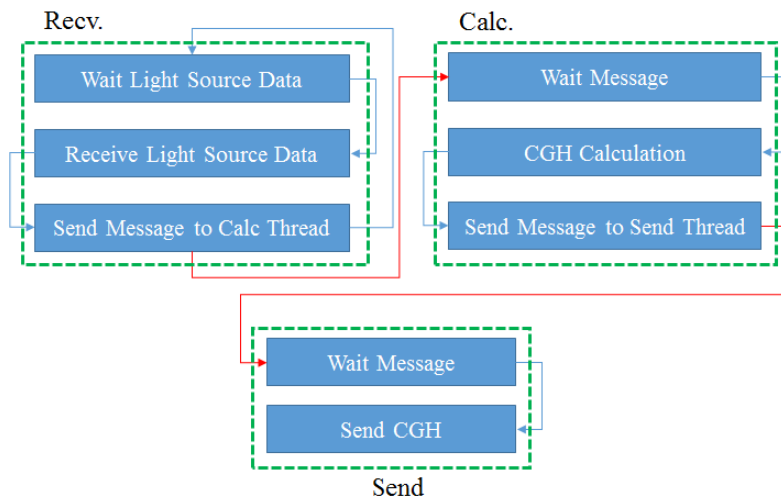
그림 4. 클라이언트 PC의 각 쓰레드에서의/사이의 프로세스 흐름 Fig. 4. Process flow in/between each thread of client PCs
