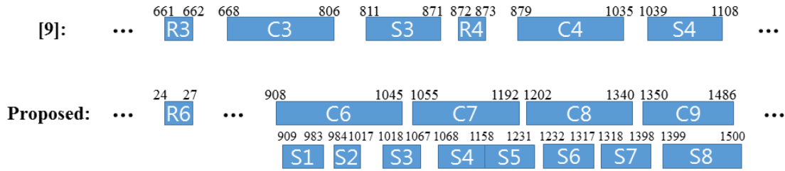
그림 5. Client_2의 각 쓰레드의 타임스탬프 다이어그램 Fig. 5. Time-stamp diagram of each thread of Client_2
