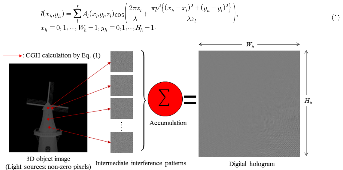
그림 1. CGH에 의한 홀로그램 생성 과정 Fig. 1. Process of generating a hologram by CGH
