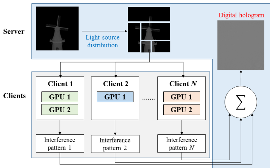
그림 2. PC 클러스터를 이용한 CGH 연산의 병렬 분산 처리
