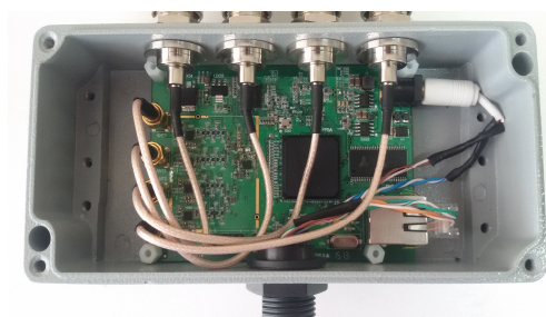
그림 2. 5.8GHz 무선모뎀
