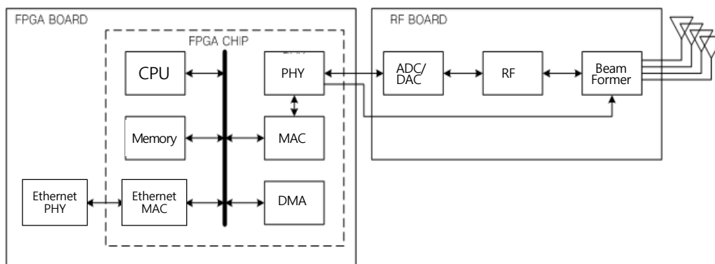
그림 1. 5.8GHz 무선모뎀 블록도
