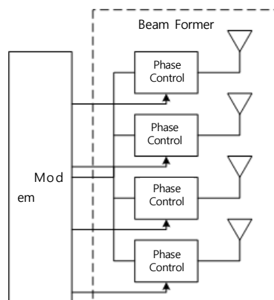
그림 3. 빔형성 블록
