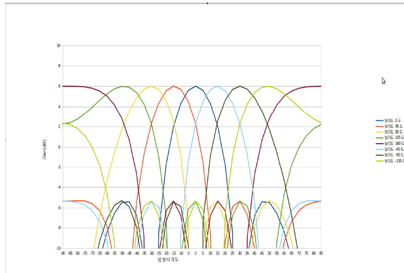
그림 4. 안테나 이득과 빔 방사각도
