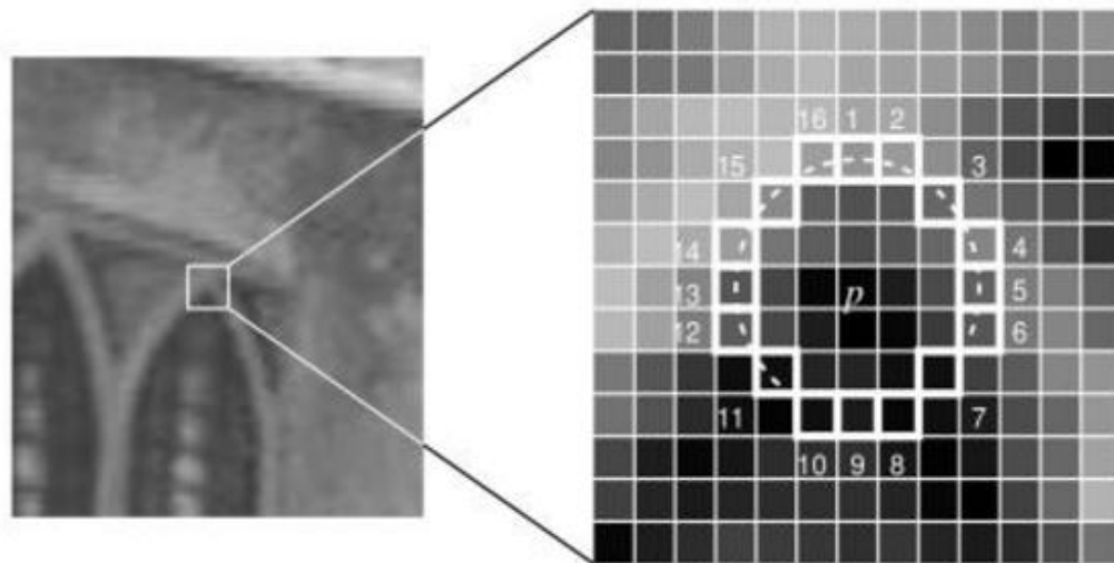
그림 2. FAST를 이용한 코너 검출 방법 (점선은 조건에 만족하는 픽셀들을 표시함)
