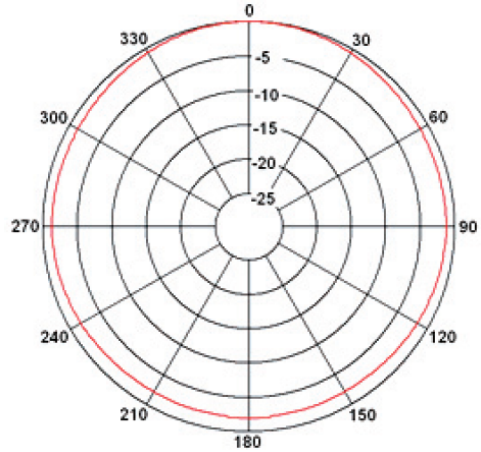
그림 4. CP-ring 안테나의 수평 방사 패턴 Fig. 4. Horizontal radiation pattern of CP-dipole antenna
