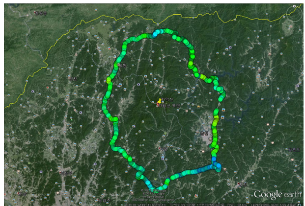
그림 8. FM 전계 강도 측정 경로(화악산) Fig. 8. FM field strength measurement route(Hwaaksan)
