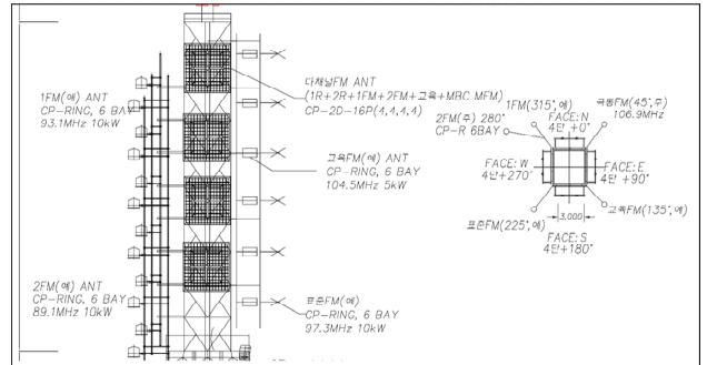
그림 5. FM 안테나(CP-dipole)설치 도면(관악산)
