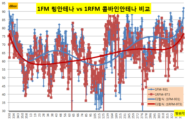
그림 7. CP-dipole 안테나와 CP-ring 안테나의 전계 강도 비교 Fig. 7. Comparison for field strength of CP-dipole antenna & CP-ring antenna
