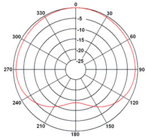
그림 10. 반사판을 가지는 CP-ring 안테나의 수평 방사 패턴 Fig. 10. Horizontal radiation pattern of CP-dipole antenna including reflector
