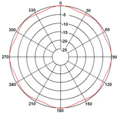
그림 2. 4방향 CP-dipole 안테나의 수평 방사 패턴 Fig. 2.. Horizontal radiation pattern of 4-Directional CP-dipole antenna
