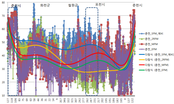
그림 9. CP-dipole 안테나와 CP-ring 안테나의 전계 강도 비교(화악산) Fig. 9. Comparison for field strength of CP-dipole antenna & CP-ring antenna(Hwaaksan)
