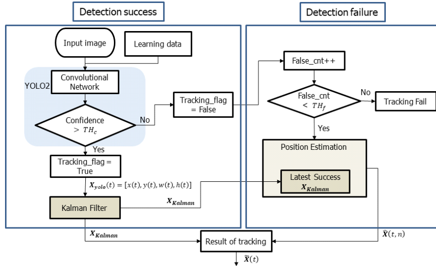
그림 3. 제안 방법의 흐름도
