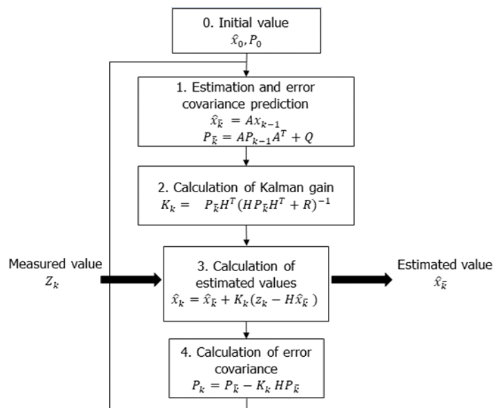
그림 1. 칼만 필터의 흐름도
