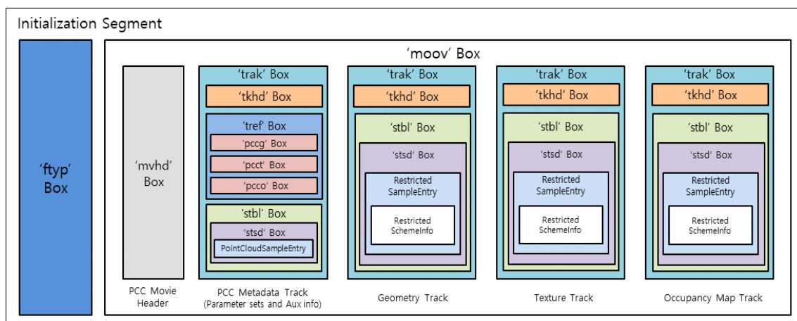
그림 4. V-PCC DASH 초기 세그먼트 구성 예시
