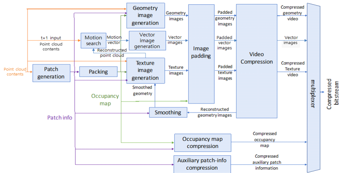
그림 1. MPEG V-PCC 부호화기
