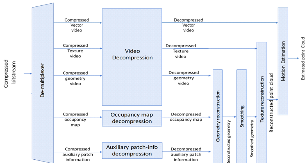
그림 2. MPEG V-PCC 복호기
