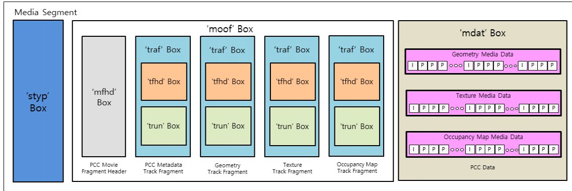
그림 5. V-PCC DASH 미디어 세그먼트 구성 예시
