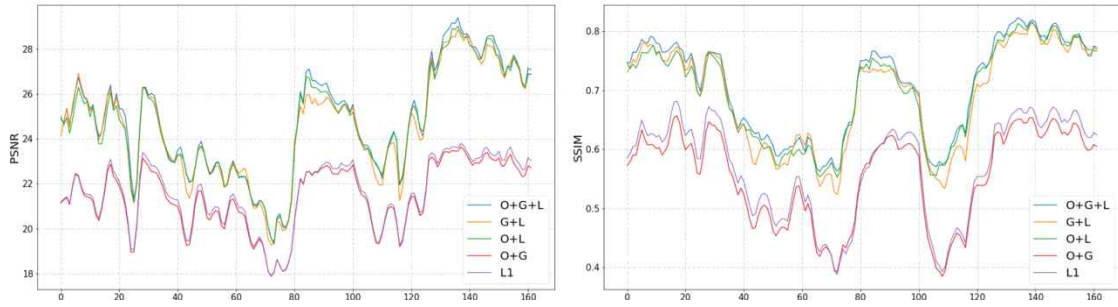
그림 7. 손실 함수에 따른 정량적 성능 비교
