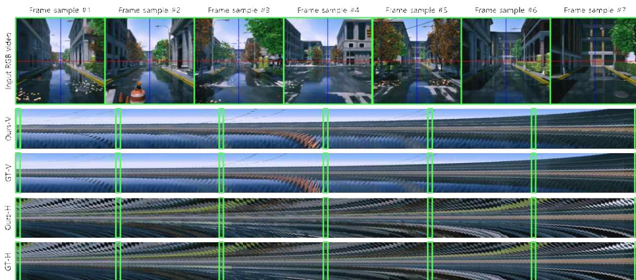
그림 4. 가상 환경 실험 영상(162 프레임)에 대한 라이트필드 비디오 합성 결과. 첫 번째 행은 입력 비디오의 샘플 프레임의 의미한다. 두 번째와 세 번째 행은 각각 제안하는 기법과 원본 영상의 수직 EPI를 시간 순서로 쌓은 결과이다. 네 번째와 다섯 번째 행은 각각 제안하는 기법과 원본 영상의 수평 EPI를 시간 순서로 쌓은 결과이다
