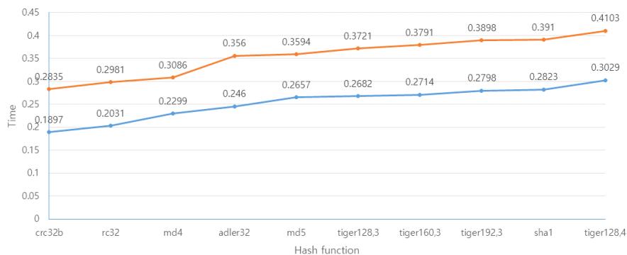
그림 4. 해시 연산 속도와 bloom필터 인덱스 생성 속도 비교
