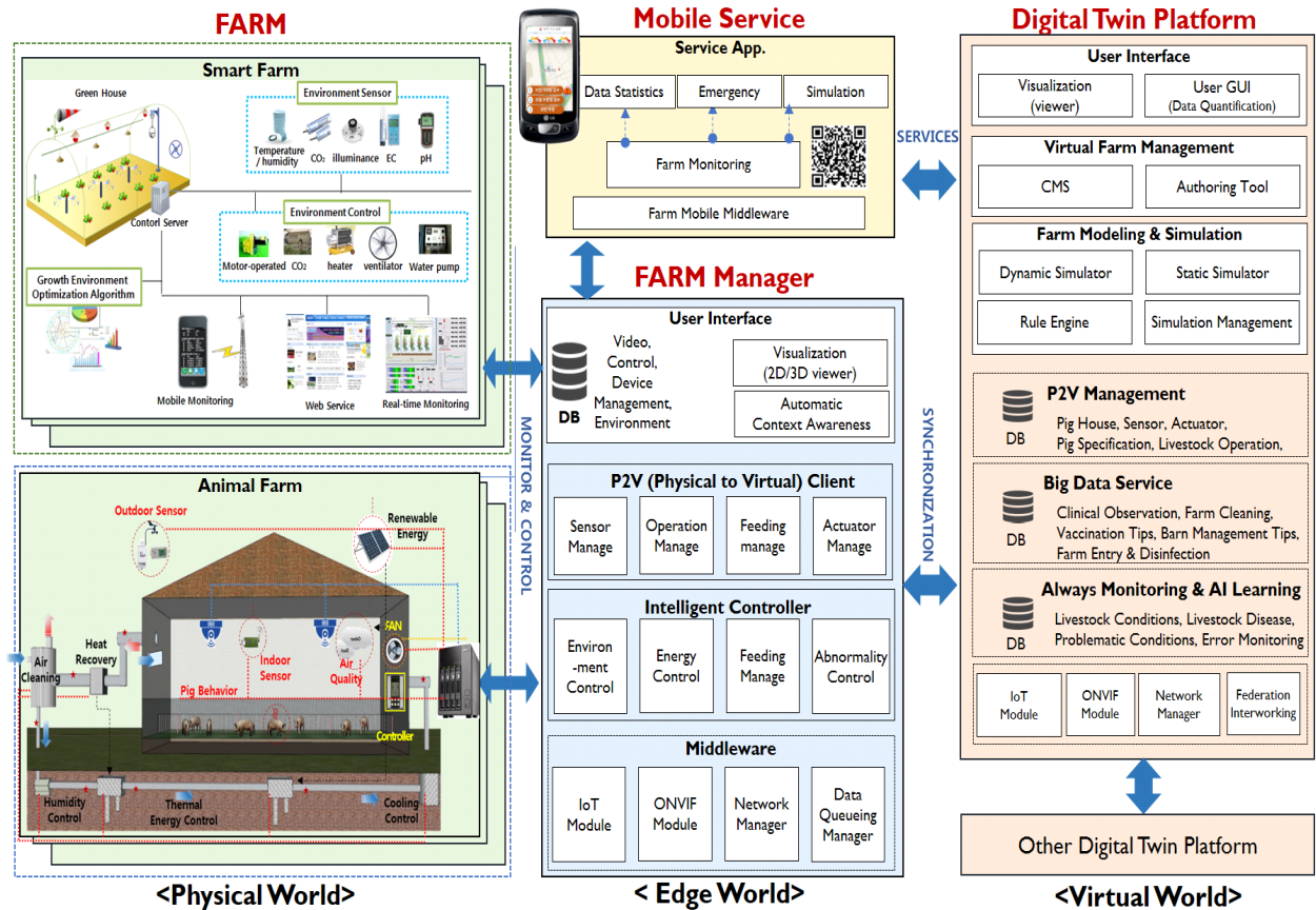
그림 4. 농·축산을 위한 계층적 디지털 트윈 아키텍처
