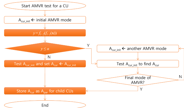
그림 1. 신경망 기반 고속 AMVR 결정 기법
