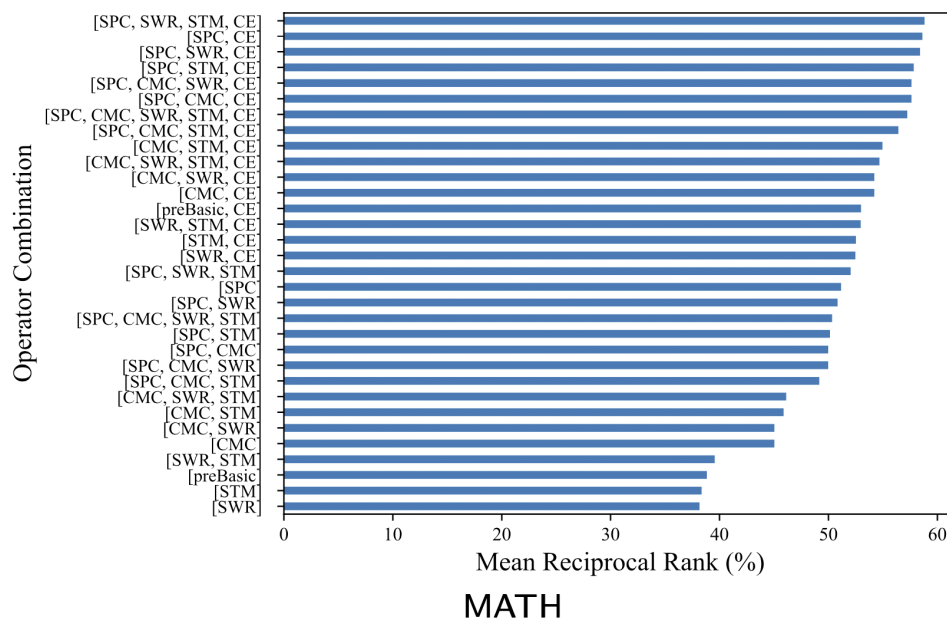
그림 1. Apache Math 프로그램에 제안된 기법을 적용한 결과
