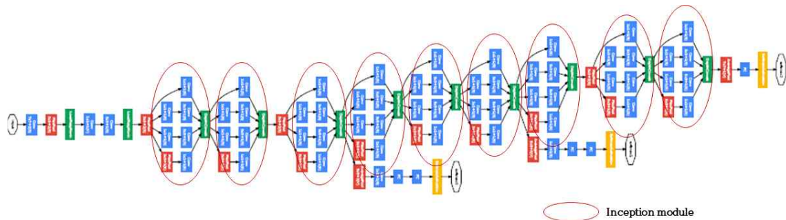
그림 8. 인셉션 모듈을 포함한 구글넷 구조
