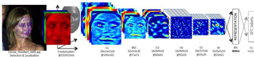
그림 1. DeepFace 네트워크 아키텍처 요약 [10]
