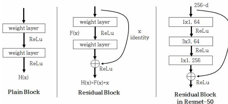
그림 9. Skip Connection을 가지는 잔차블록
