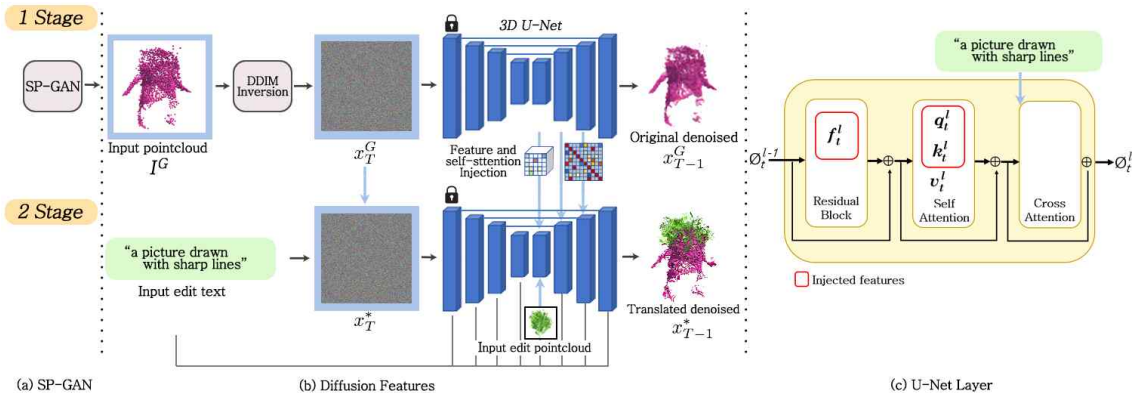
그림 8. 포인트 클라우드를 창의적으로 생성하기 위해 우리가 제안하는 방법(SP-GAN->Diffusion model+CLIP) Fig. 8. How we propose to creatively create a point cloud(SP-GAN->Diffusion model+CLIP)
