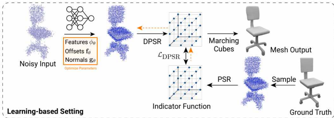
그림 16. 학습 기반 표면 재구성을 위한 파이프라인 Fig. 16. Pipeline for learning-based surface reconstruction
