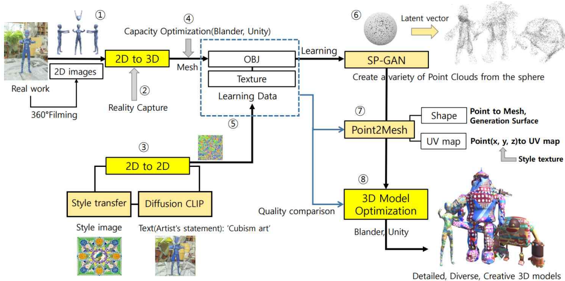
그림 2. 2D to 3D 창의적 생성을 위한 실험 Fig. 2. Experiments for 2D to 3D Creative Generation
