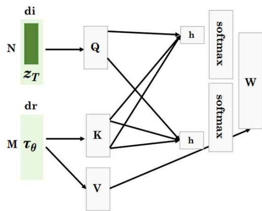
그림 11. Cross Attention 작동모습 Fig. 11. Cross Attention operation
