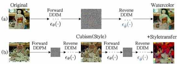
그림 5. 2D to 2D 스타일 텍스처 생성 과정 Fig. 5. Process for creating 2D to 2D style textures
