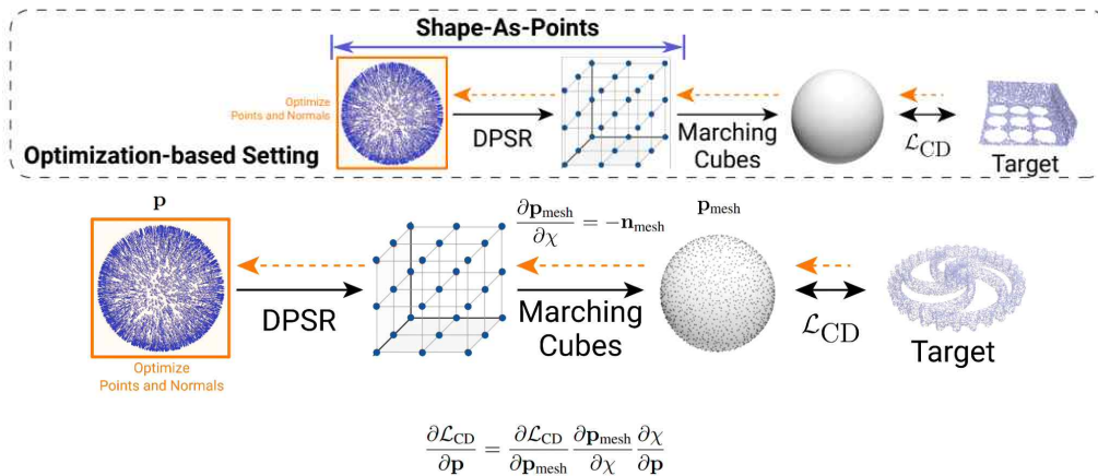
그림 14. SAP 최적화 기반 3D 재구성 Fig. 14. SAP Optimization-based Setting
