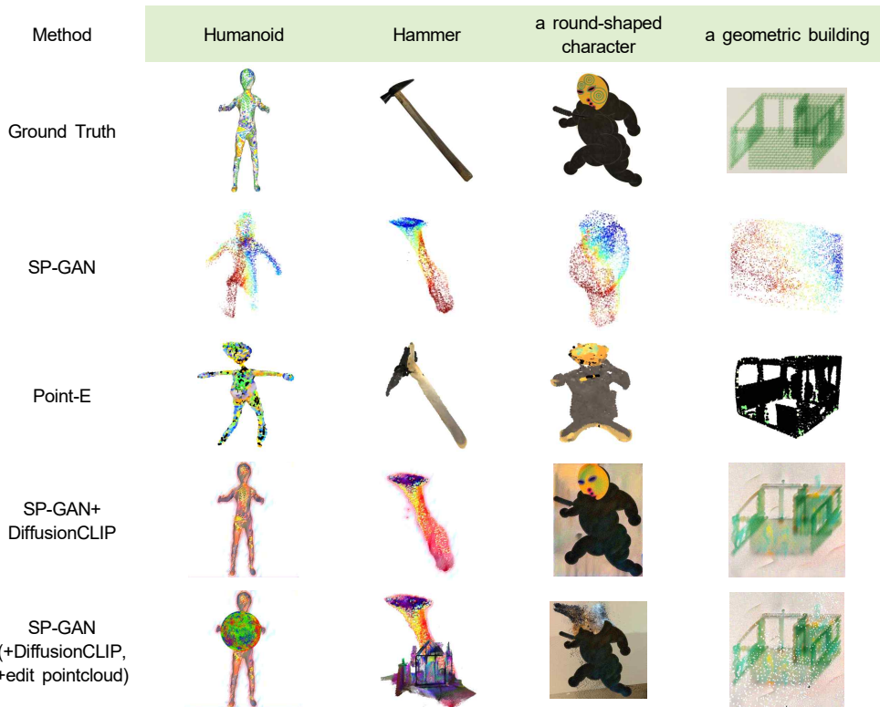
그림 13. 3D로부터 다양한 포인트 클라우드 생성 비교 Fig. 13. Comparison of creating different point clouds from 3D
