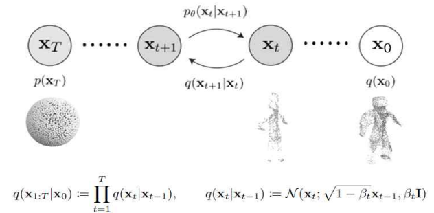
그림 9. 확산 및 생성 프로세스의 시각화. 순방향 전이 확률 q(x_t|x_{t+1}, x_0) 이후 p_\Theta(x_t|x_{t+1}) 를 학습할 수 있다.
