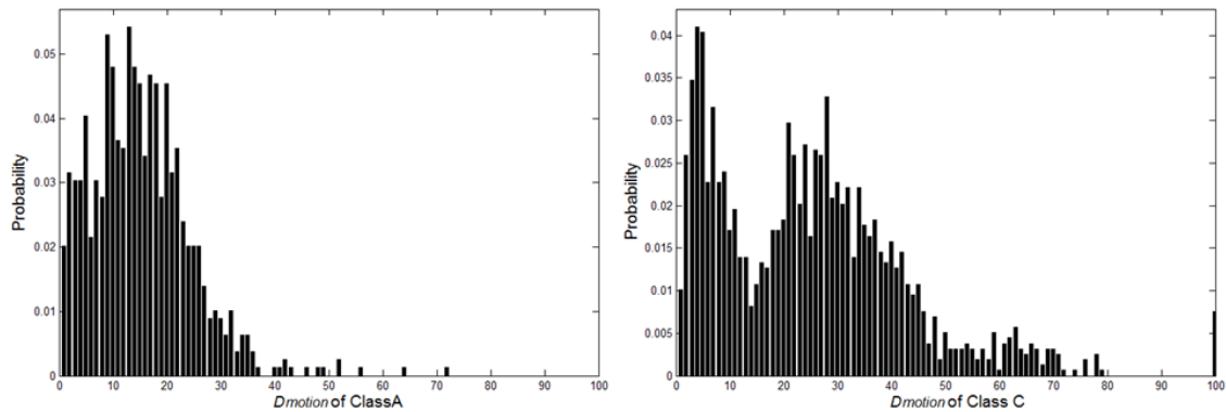
그림 11. Class A와 C 영상의 D_{motion} 분포들
