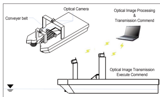
〈그림 3〉 해양 부유물 수거용 수상드론
