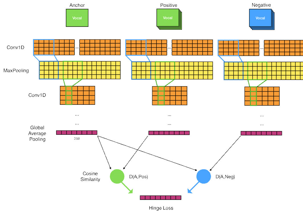
그림 5. 가수 인식 네트워크 구조 (거리 기반 학습)
