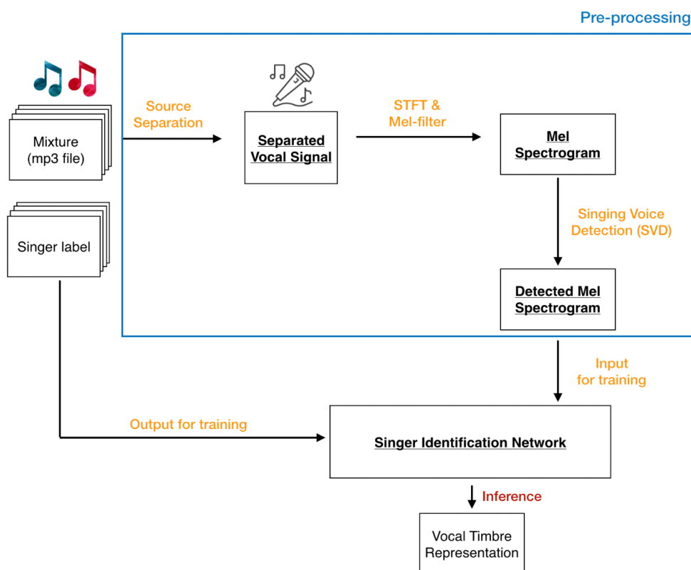
그림 1. 음색기반 음악 특성 추출에 관한 전체 개요도
