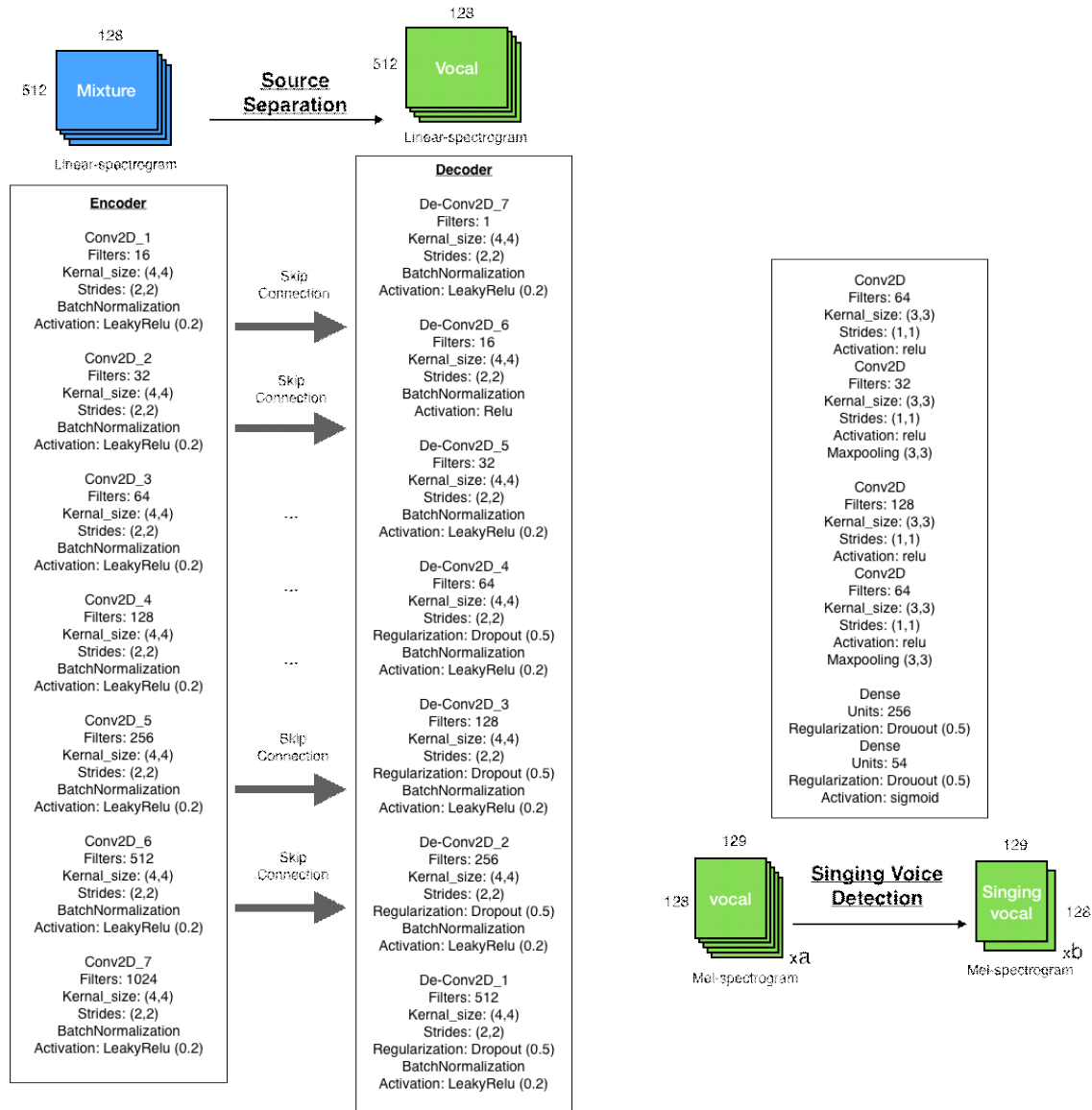
그림 2. 보컬 분리 모델 및 보컬 등장구간 추출 모델 상세
