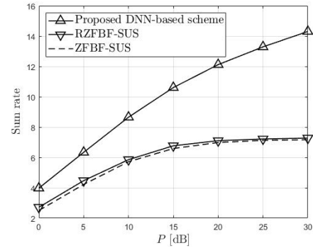
그림 2. 송신 파워 vs. Sum rate
